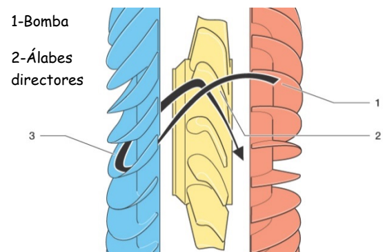
Fig. 17 Detalle interno del convertidor
