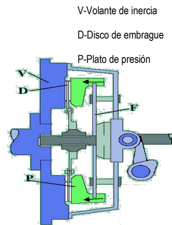
Fig. 7 Embragado
